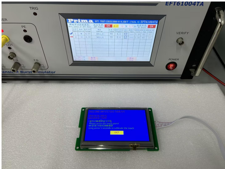
图 5-4 群脉冲测试图
