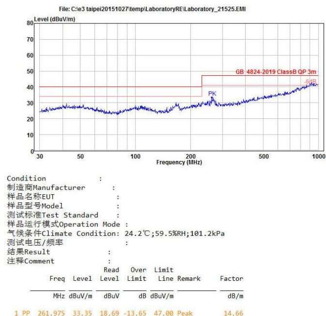
图 5-6 辐射测试水平方向
