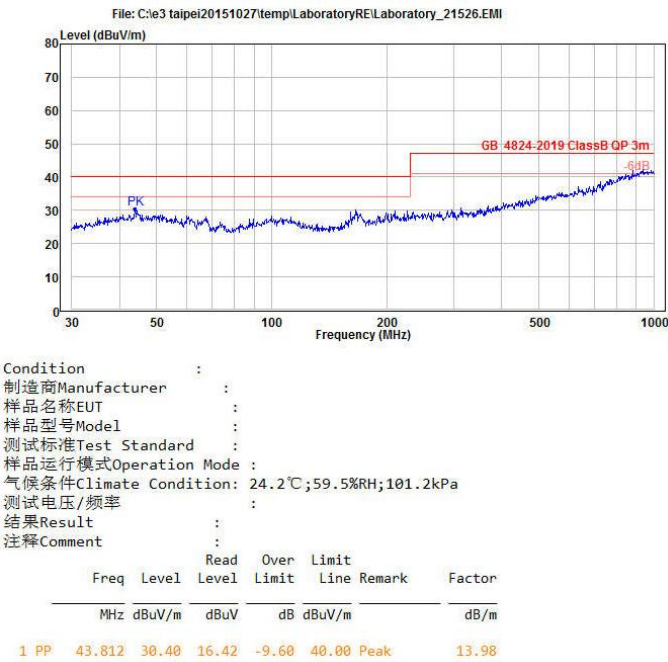
图 5-7 辐射测试垂直方向
